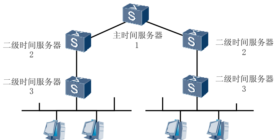
图 4-1 NTP 网络结构
