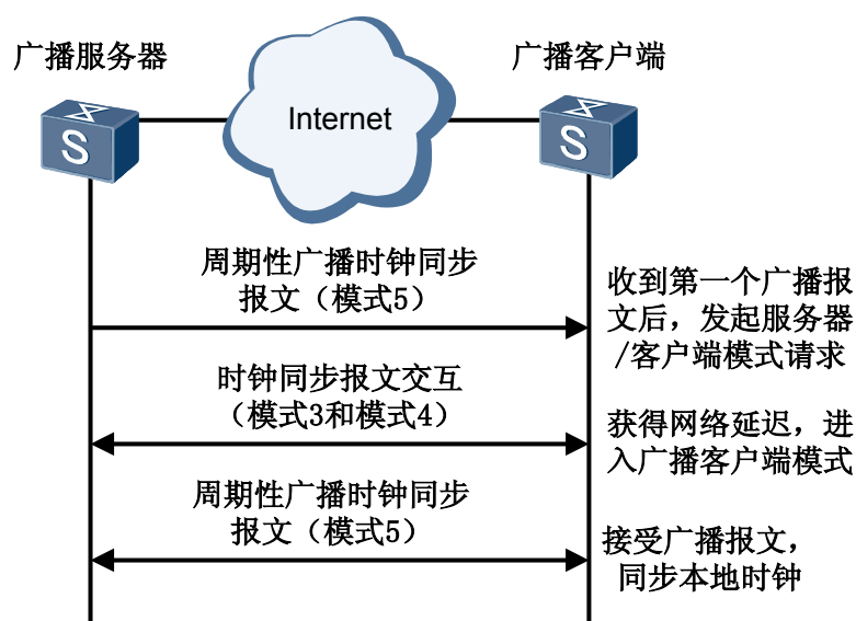
图 4-4 广播模式
