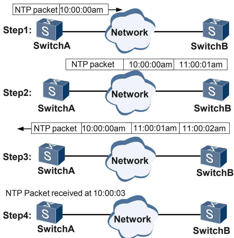
图 4-6 NTP 实现过程图
