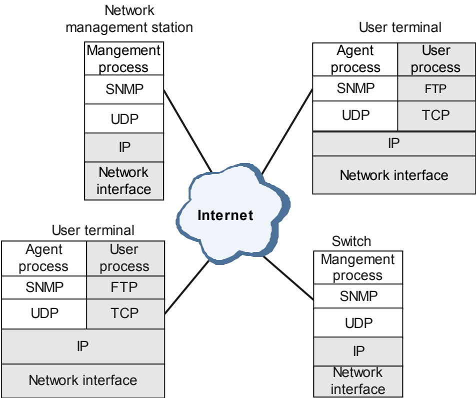
图 1-1 SNMP 典型配置
