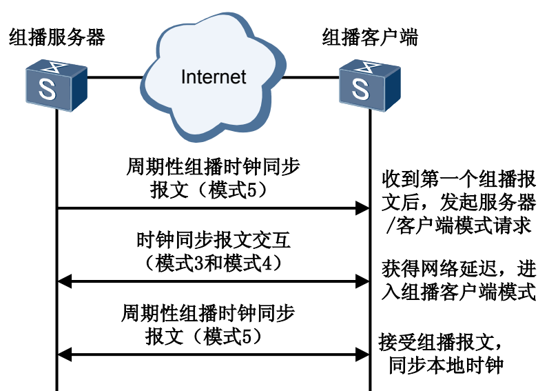
图 4-5 组播模式
