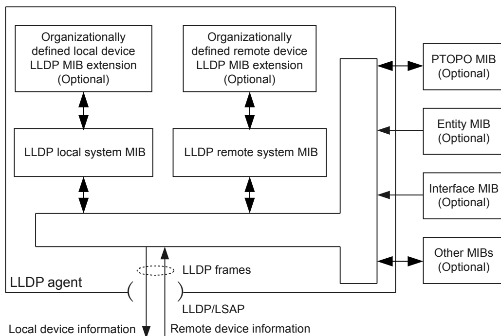
图 2-4 LLDP 结果框图
