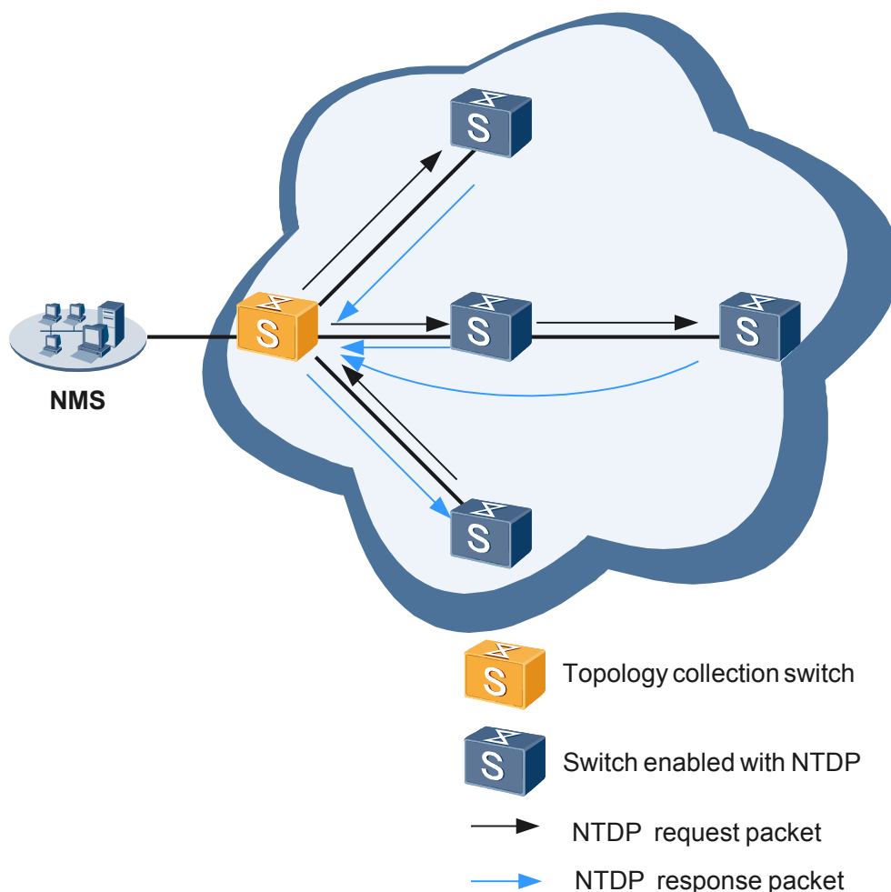
图 6-3 NTDP 拓扑信息收集示意图
