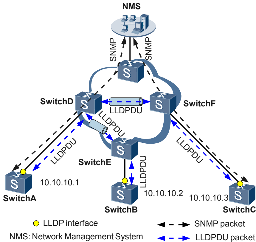
图 2-6 多邻居组网方式
