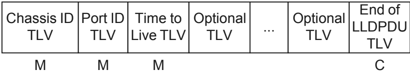
图 2-2 LLDPDU 结构图
