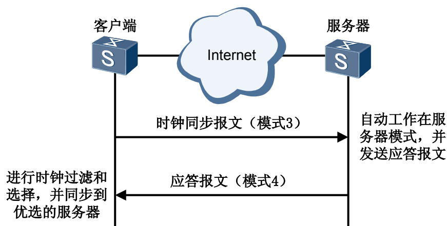
图 4-2 客户/服务器模式
