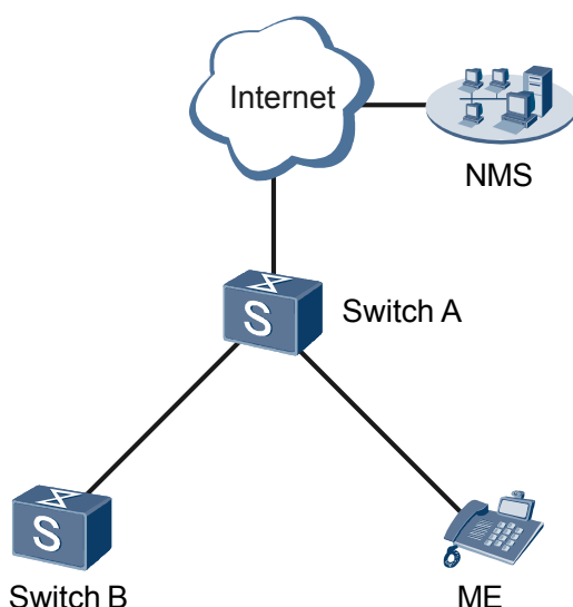
图 2-5 单邻居组网方式
