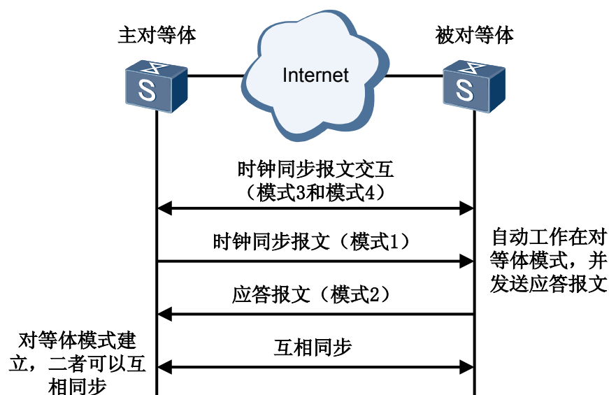
图 4-3 对等体模式
