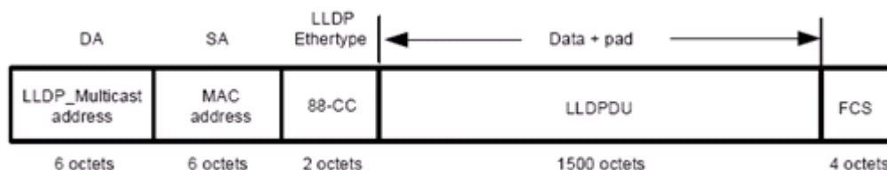
图 2-1 LLDP 报文结构
