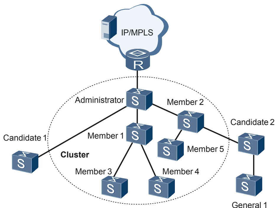
图 6-4 HGMP 的应用
