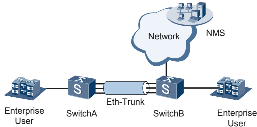
图 2-7 存在链路聚合的组网方式
