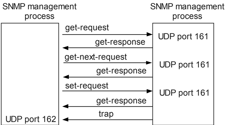
图 1-4 SNMP 的报文操作
